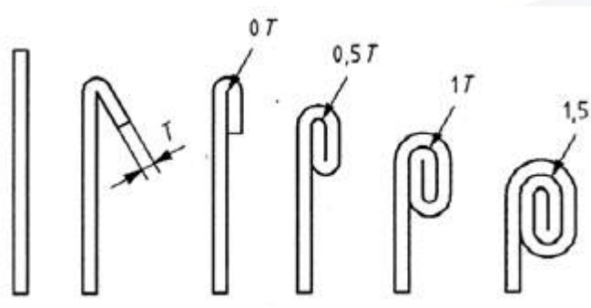
Figure 9 - T-bends
